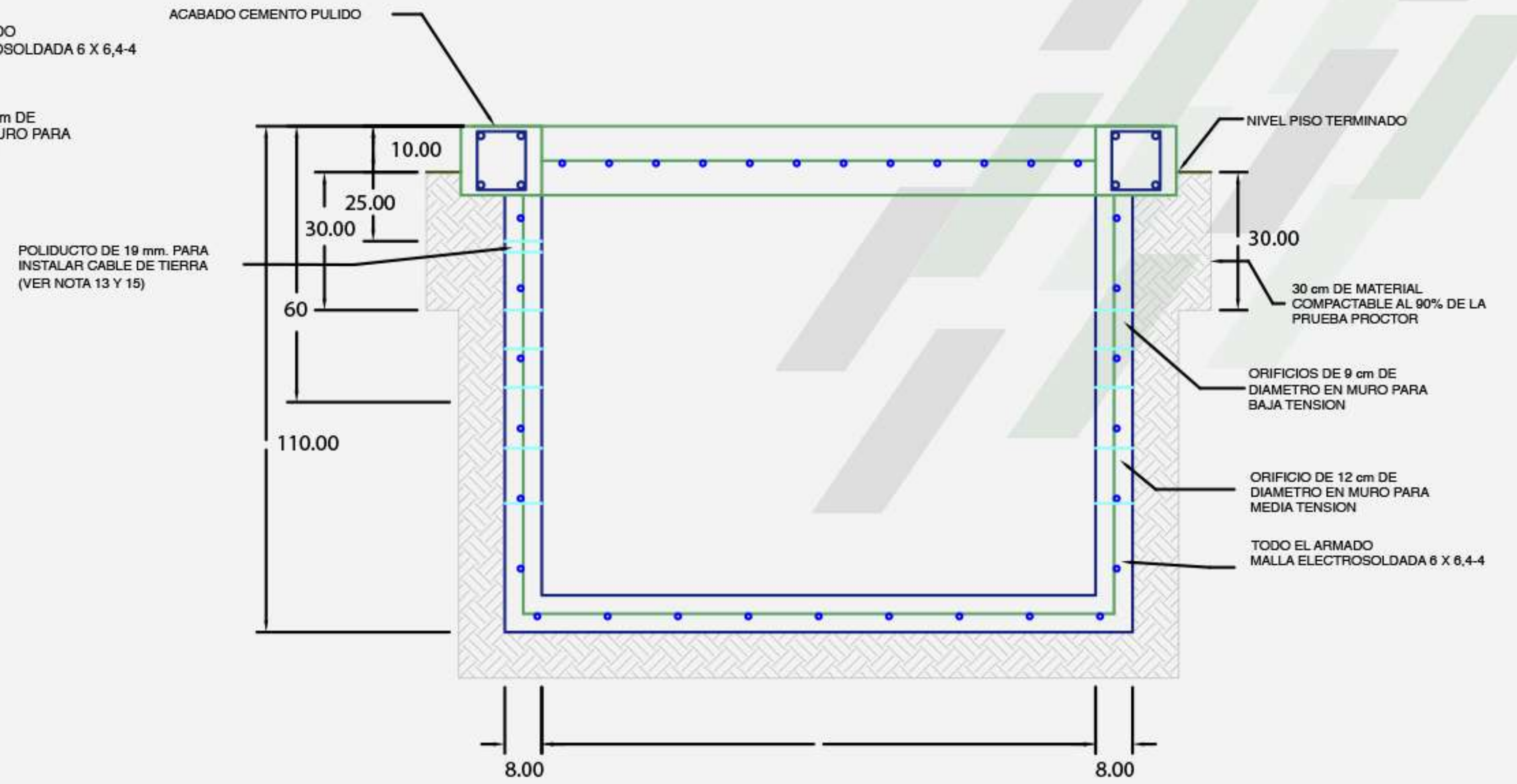
NIVEL FREÁTICO ALTO CORTE B-B'
